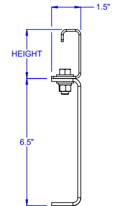
OPTIONAL GUARDRAIL
