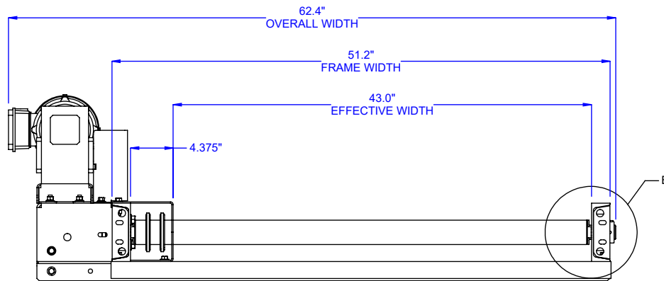
VIEW A-A
