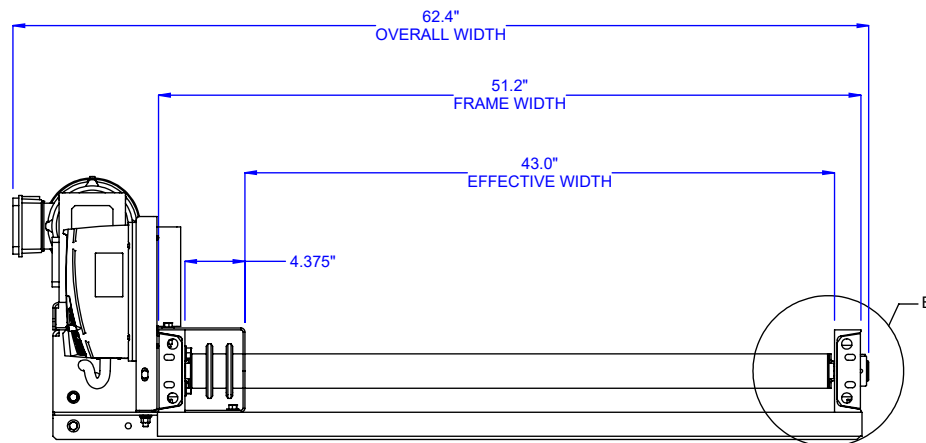
VIEW A-A
