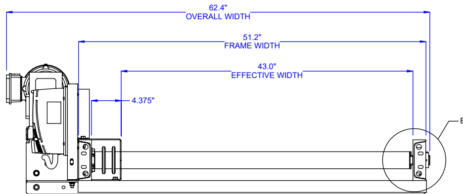
VIEW A-A
