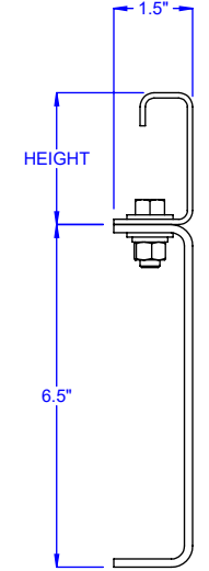
OPTIONAL GUARDRAIL
