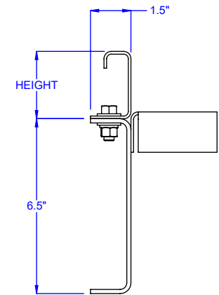
OPTIONAL GUARDRAIL
